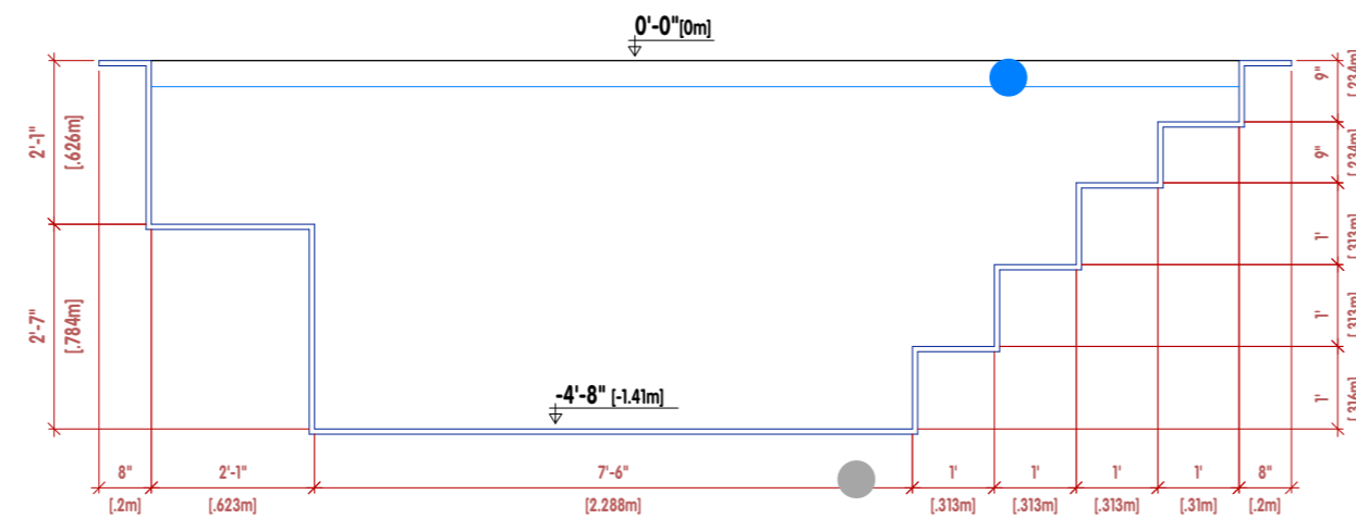
LONGITUDINAL SECTION A-A
