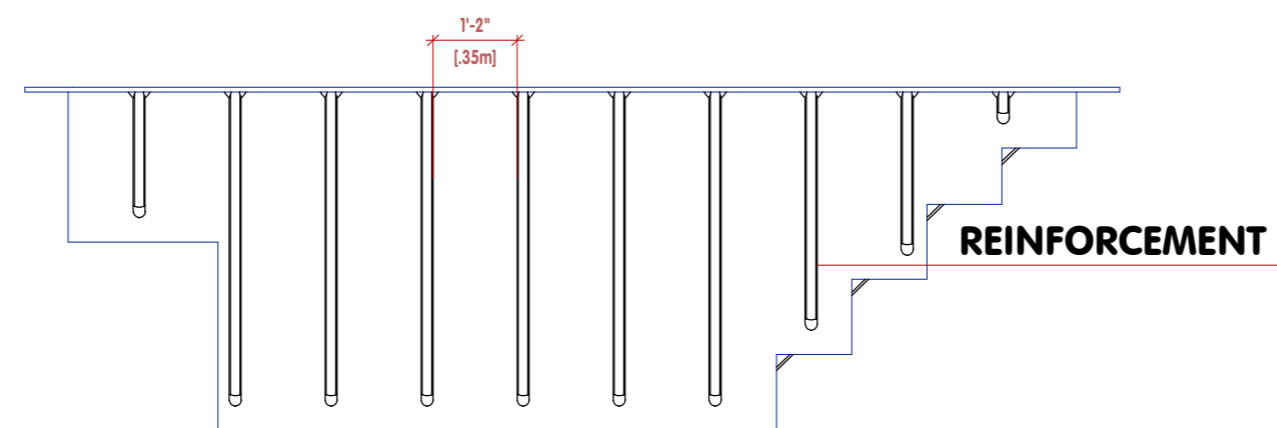
LONGITUDINAL SIDE VIEW C-C
