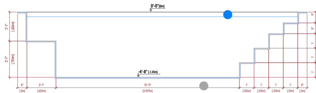
LONGITUDINAL SECTION A-A
